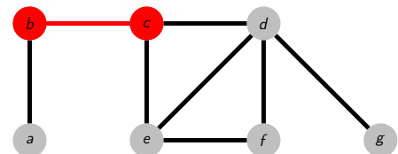
выбираем ребро (b, c)
