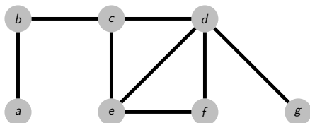
дан граф на семи вершинах
