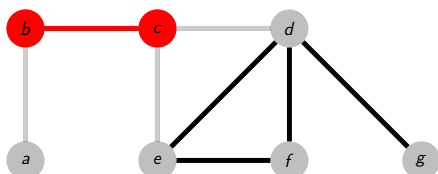
покрытые ребра удаляем
