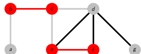
выбираем ребро (e, f)
