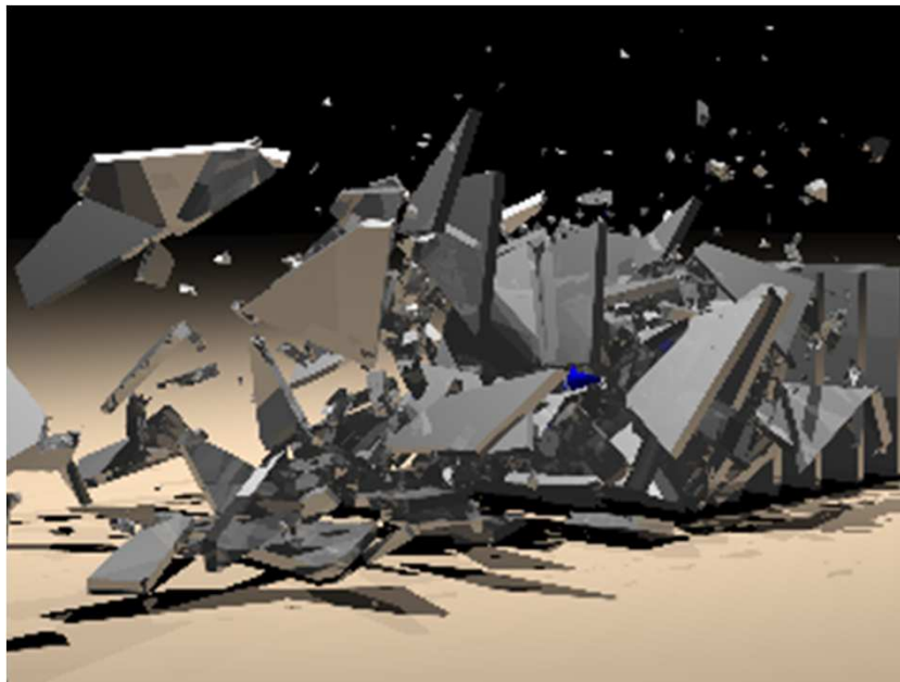
Рис. 6. Fedkiw
