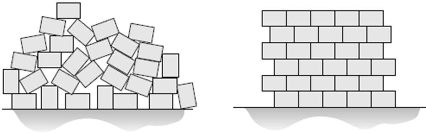
Рис. 10. Erleben
