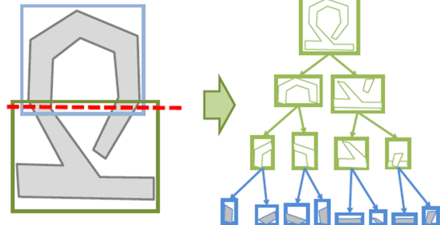
Рис. 20, Coumans
