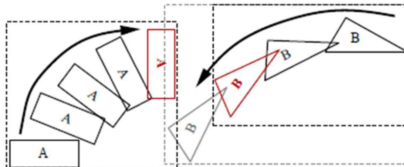
Рис. 13. Mirtich
