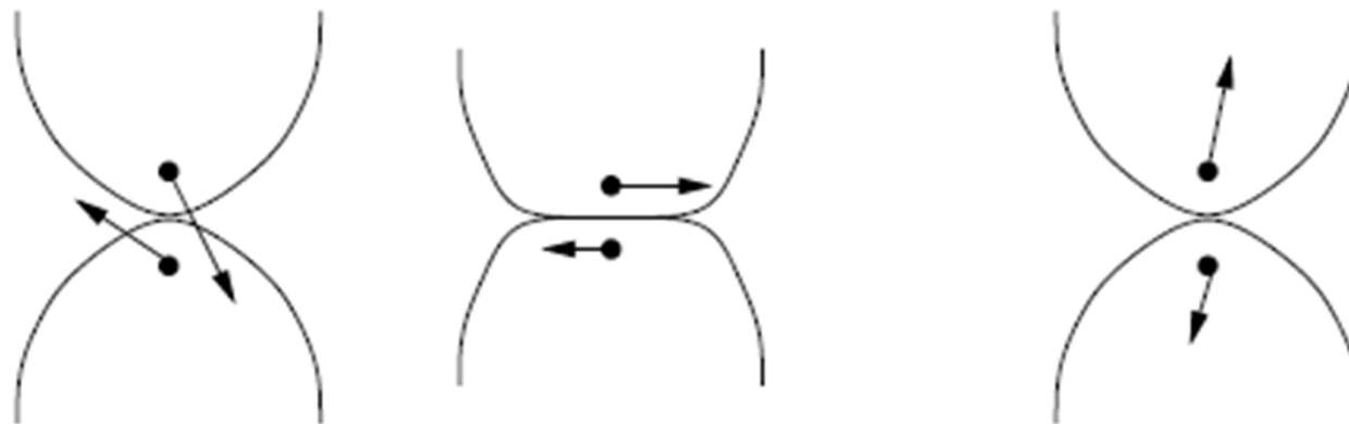
Рис. 9. Mirtich, Canny
