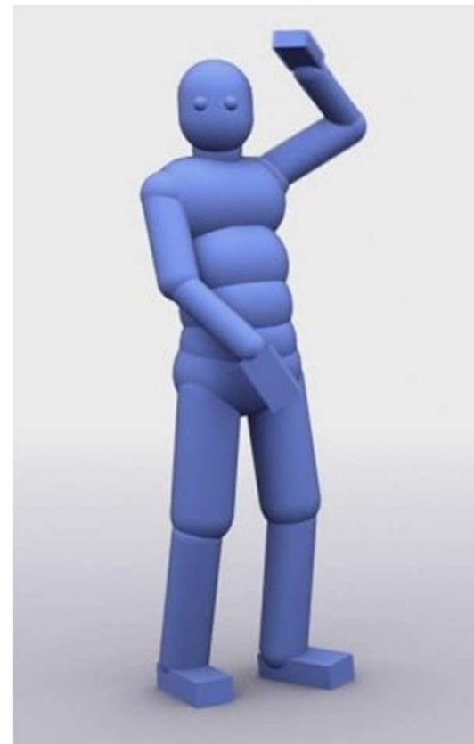
Рис. 14. Naturalmotion
