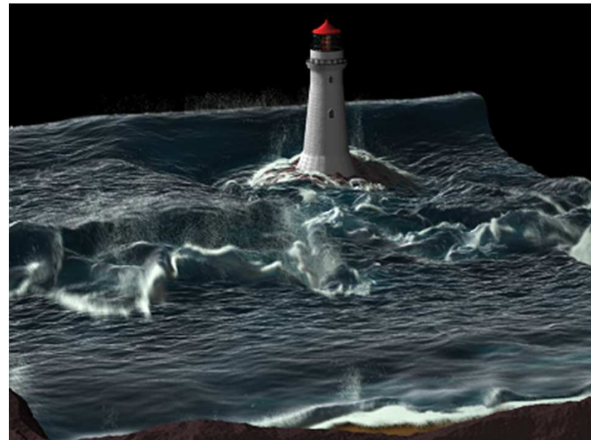
Рис. 7. Fedkiw
