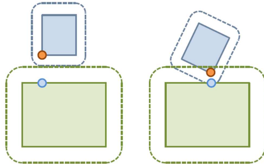
Рис. 15. Coumans
