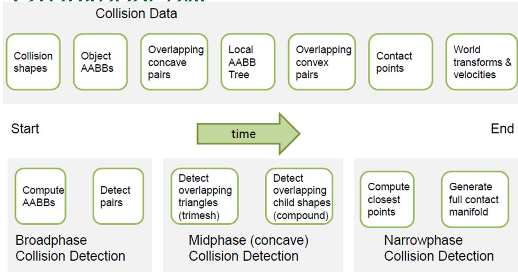
Рис. 21, Coumans
