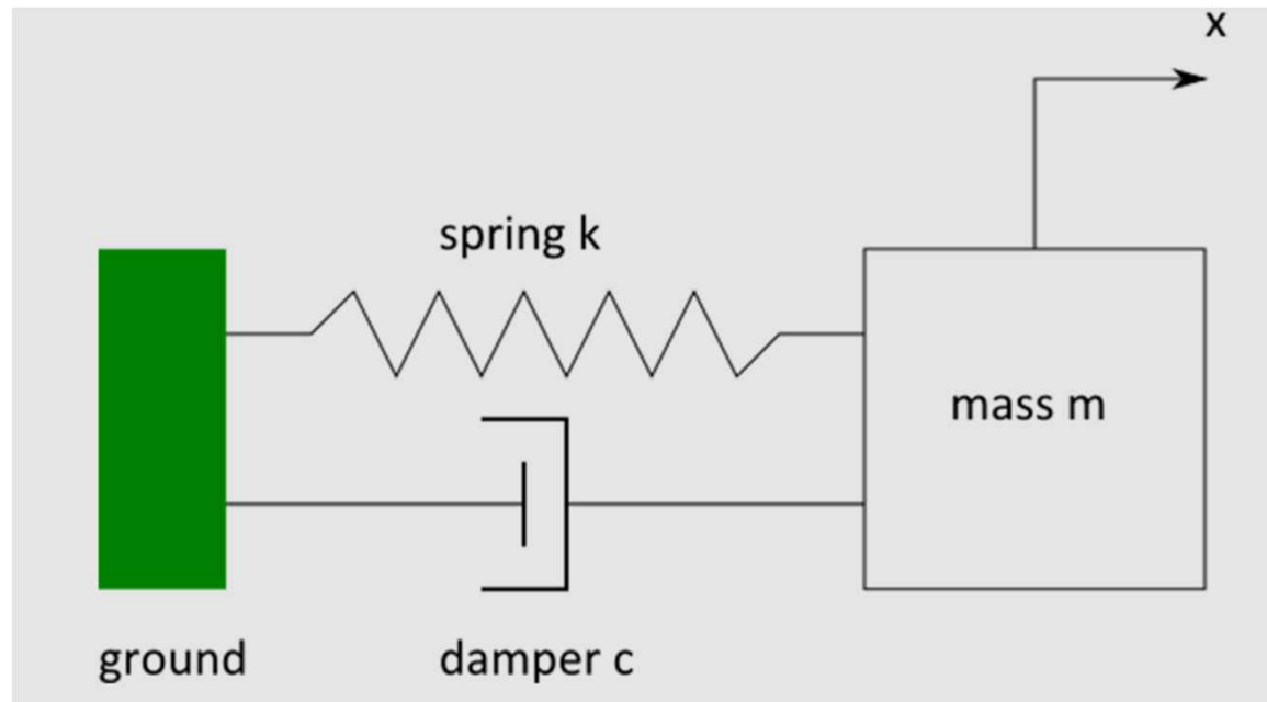
Рис. 12. Catto
